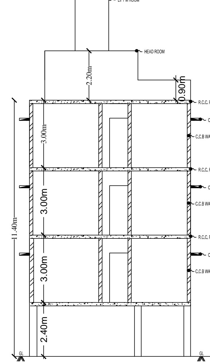
SECTION @A-A'
